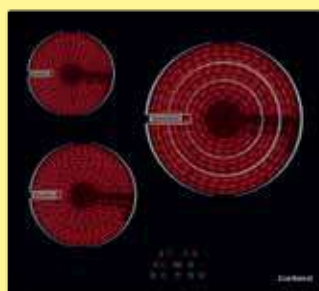
VITROCERAMICA TOUCH CONTROL BISELADA CCVG-3BL574 • Medidas ext.: 59x52 • Medida encastre: 56X49
