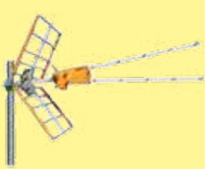
ANTENA EXTERIOR mod. ZENIT • Ganancia 15db • Canales del 21 al 48 Rf. 149222
